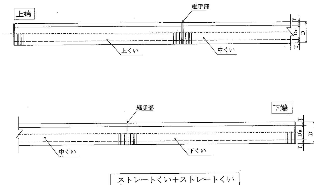
図 I-3-1 標準形状図
